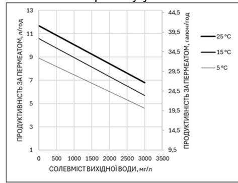
Продуктивність по пермеату установки Ecosoft MO6
