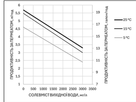
Продуктивність по пермеату установки Ecosoft MO3
