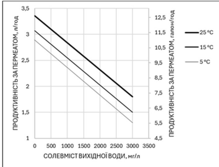
Продуктивність по пермеату установки Ecosoft MO2
