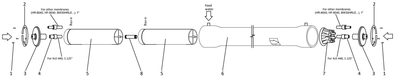
1 – гвинти, 2 – фіксуючі елементи, 3 – торцева кришка, 4 – адаптер, 5 – мембрана, 6 – мембранотримач, 7 – упорне кільце, 8 – з'єднуючий елемент для мембран
