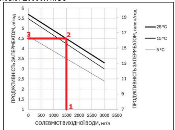
Продуктивність по пермеату установки Ecosoft MO9
