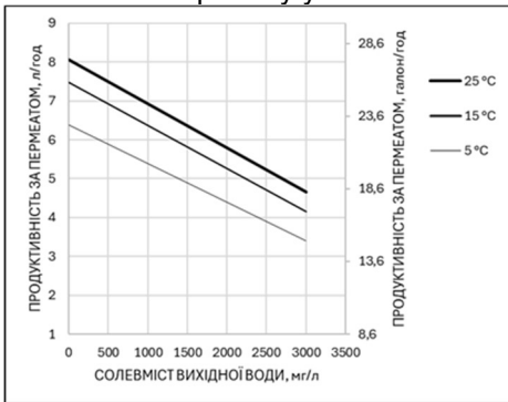
Продуктивність по пермеату установки Ecosoft MO4
