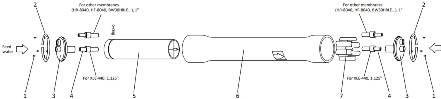
1 – гвинти, 2 – фіксуючі елементи, 3 – торцева кришка, 4 – адаптер, 5 – мембрана, 6 – мембранотримач, 7 – упорне кільце
