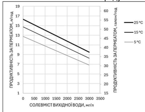
Продуктивність по пермеату установки Ecosoft MO9
